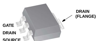
SOT-223
