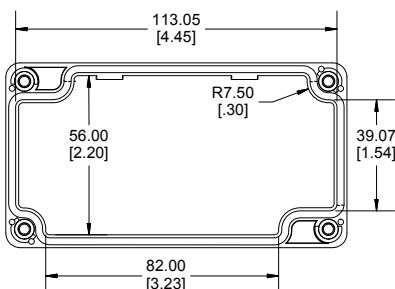
INSIDE LID
