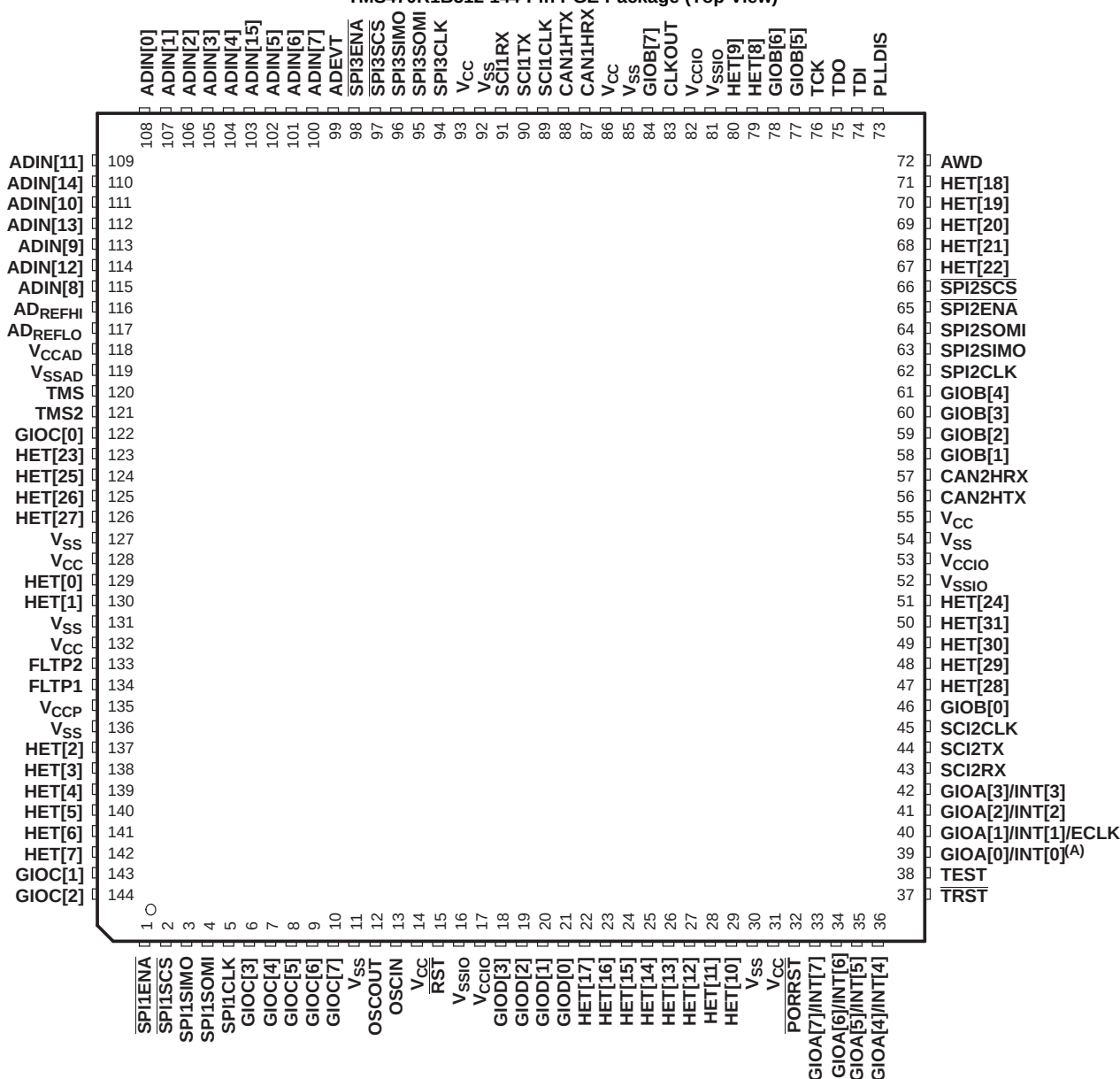
TMS470R1B512 144-Pin PGE Package (Top View)
