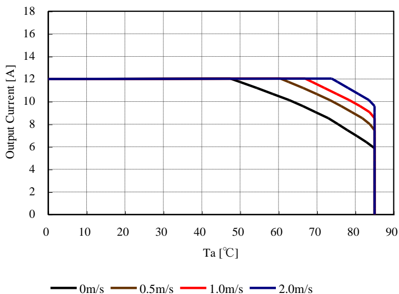
MPDRX104S Thermal Derating
