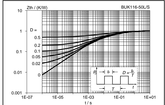
Fig. 7. Transient thermal impedance. Z_{th\ j-mb} = f(t) ; parameter D = t_b/T
