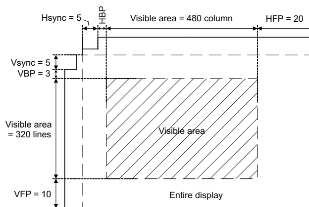
Figure 23. HVGA Display Parameters
