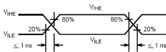
(d) ECL Input Test Waveform
