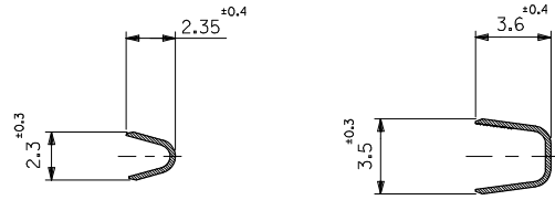
断面 A-A SECT.A-A
