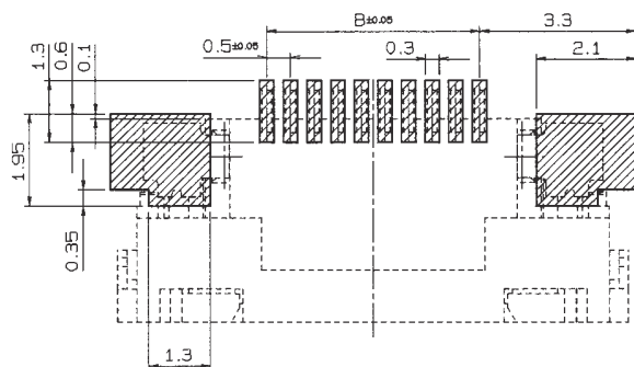
推奨取り付け寸法 (コネクタ搭載側)
