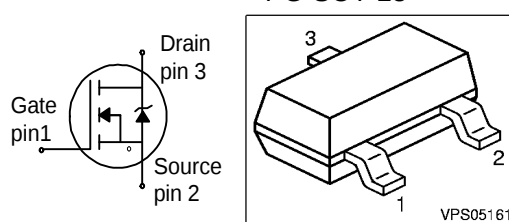
PG-SOT-23
