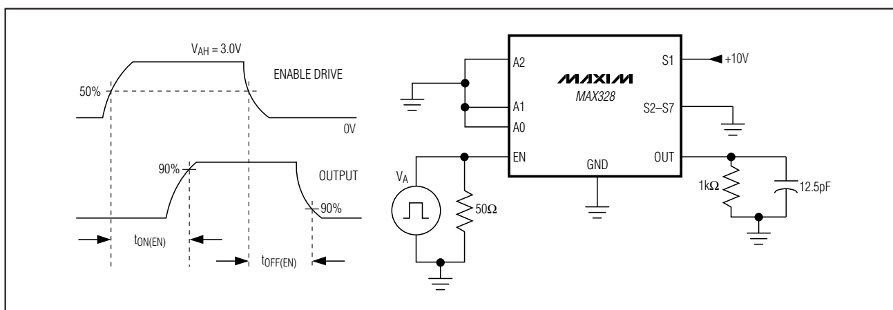
Figure 3. Enable Delay ( t_{ON(EN)} , t_{OFF(EN)} )
