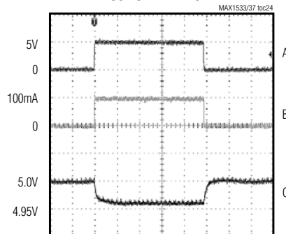
LDO5 LOAD TRANSIENT
