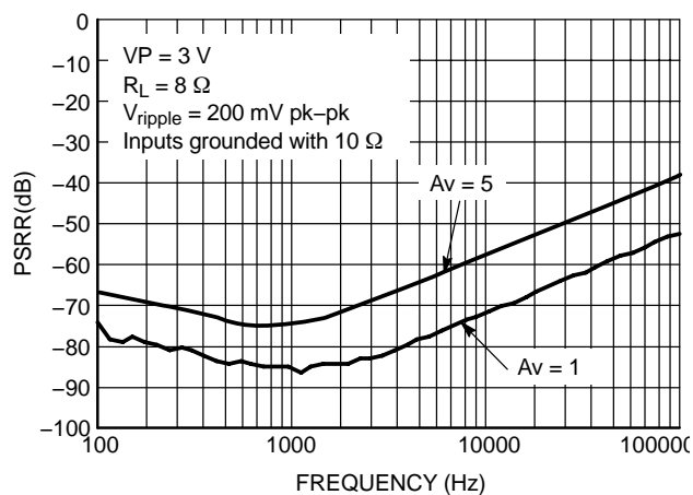
Figure 15. PSRR versus Av @ VP = 3 V
