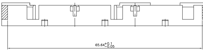
SECTION A-A
