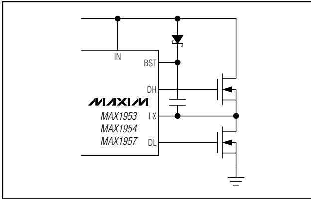
Figure 5. DH Boost Circuit
