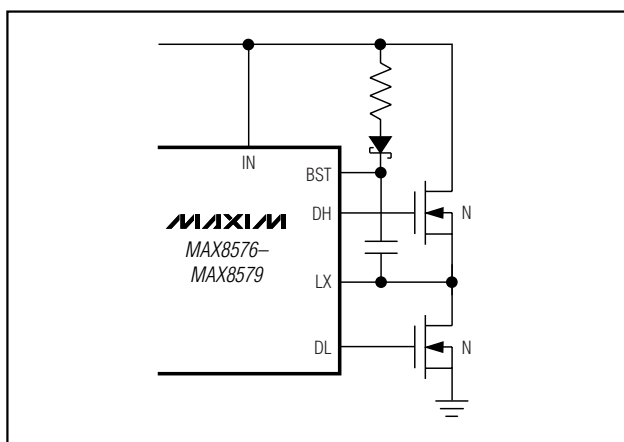
Figure 4. DH Boost Circuit
