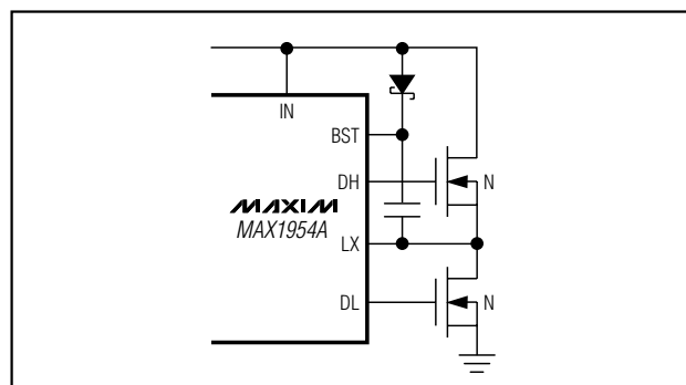
Figure 3. DH Boost Circuit
