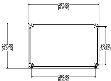
BOTTOM OF LID
