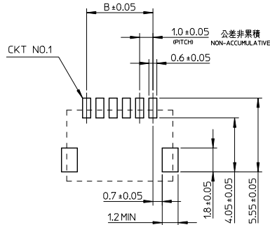
参考パターンレイアウト RECOMMENDED PATTERN (DRUREP) SCALE:5-1
