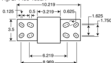
Fig. 2: 1400-1600A
