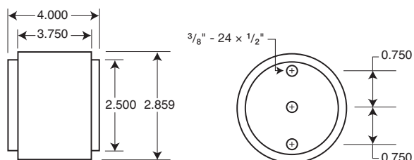
Fig. 3: 800A
