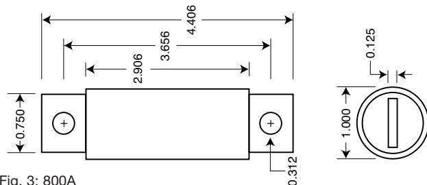
Fig. 3: 800A
