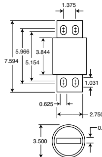
Fig. 2: 900-1000A
