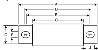
Fig. 2: 1400-1600A
