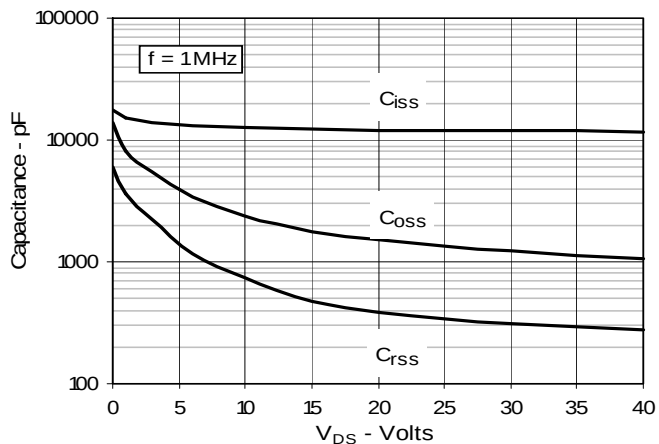
Fig. 11. Capacitance
