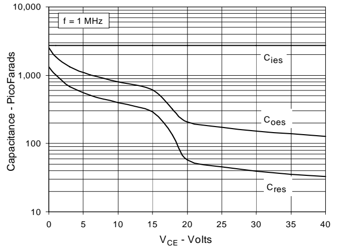
Fig. 16. Capacitance
