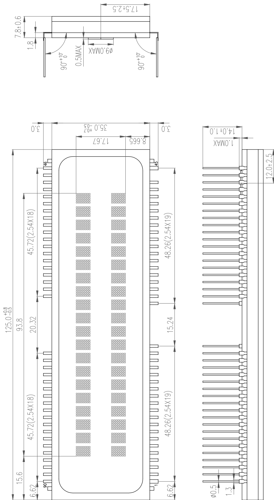
附图 1: 外形图 (Unit:mm)
