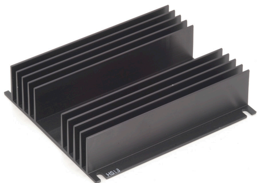
HS13 1.48°C/W
