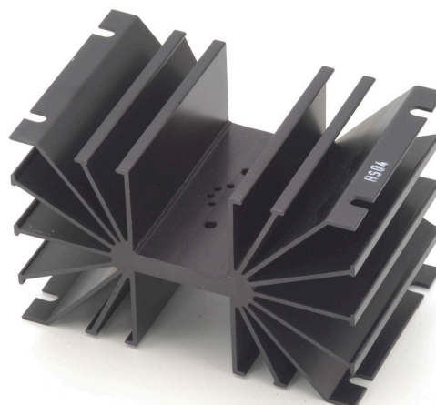
HS04 0.95°C/W
