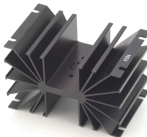
HS04 0.95°C/W
