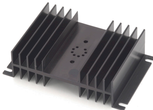
HS03 1.7°C/W
