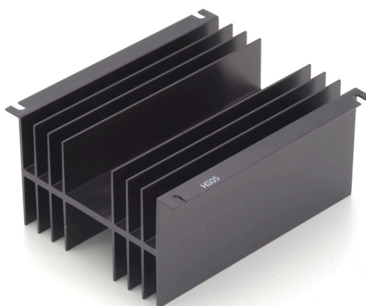
HS05 0.85°C/W
