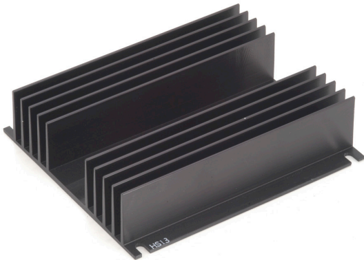
HS13 1.48°C/W
