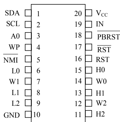
20-Pin TSSOP
