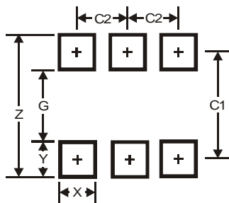
SOT563
