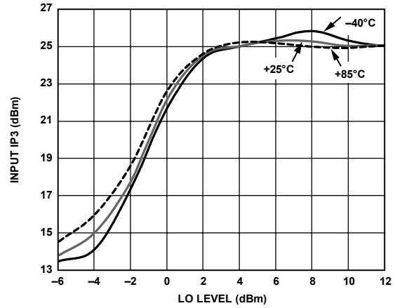
Figure 24. Input IP3 vs. LO Level
