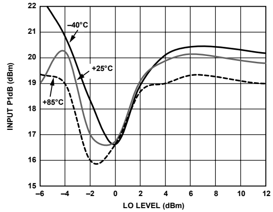
Figure 25. Input P1dB vs. LO Level
