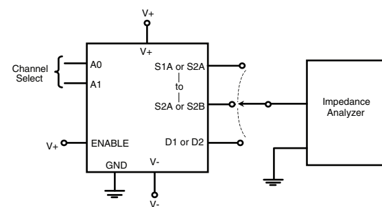
Fig. 8 - Source/Drain Capacitance
