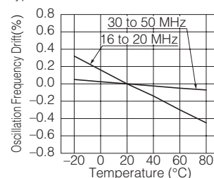
Type EFOJM
