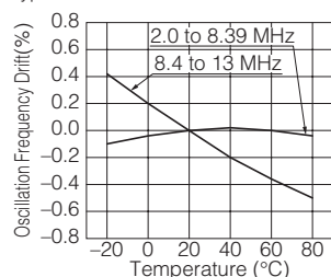
Type EFOSM
