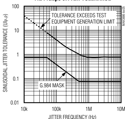
1.244Gbps JITTER TOLERANCE
