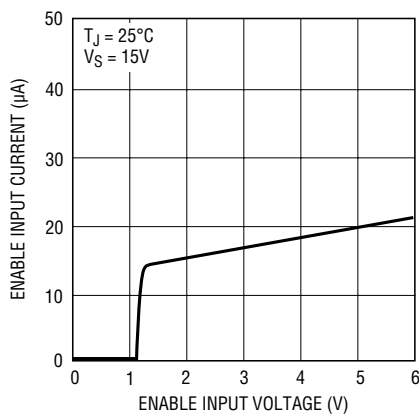
Enable Input Current
