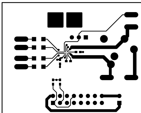
Figure 30. Top Layer
