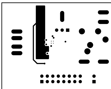
Figure 32. Layer 3 (V DD )
