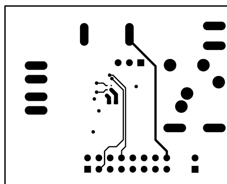
Figure 33. Bottom Layer
