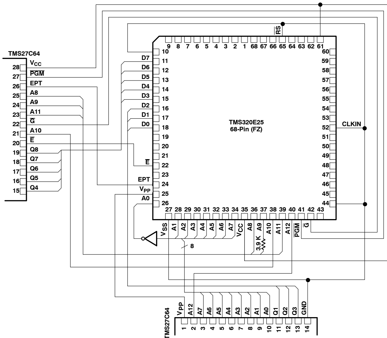
Pin Nomenclature (TMS320E25)
