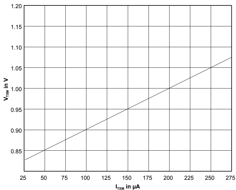
V_{TXM} vs I_{TXM}
