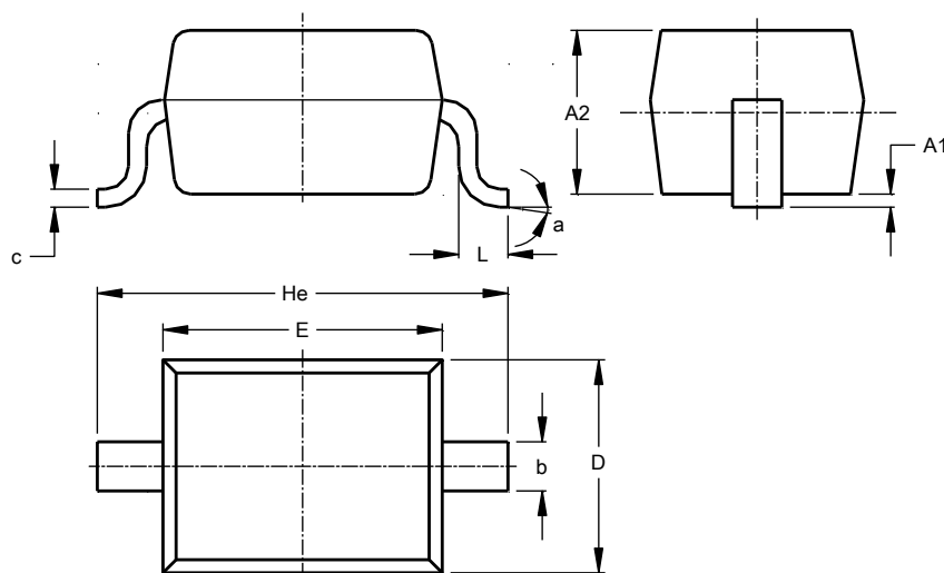
SOD323
