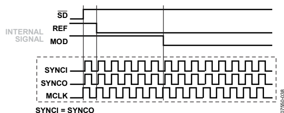
Figure 38. SYNCI = SYNCO
