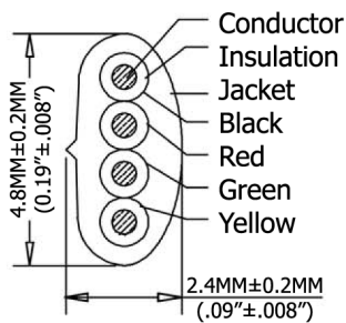
SEC:A-A
