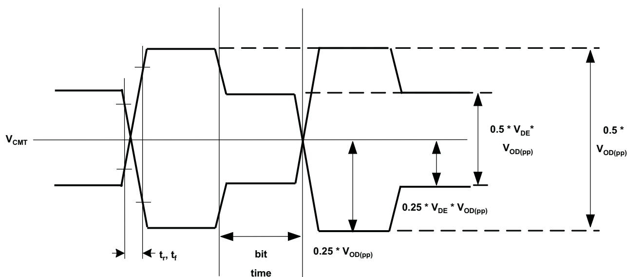
Figure 4-1. Transmit Output Waveform Parameter Definitions
