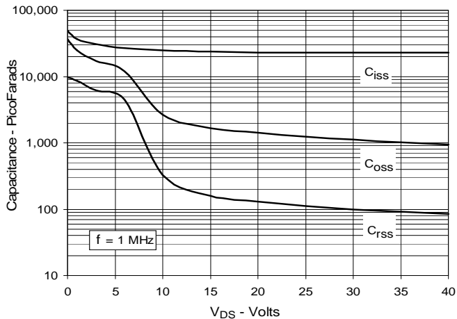
Fig. 11. Capacitance
