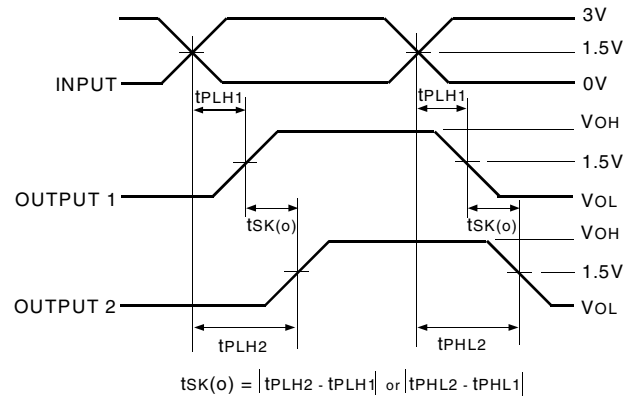
Output Skew
