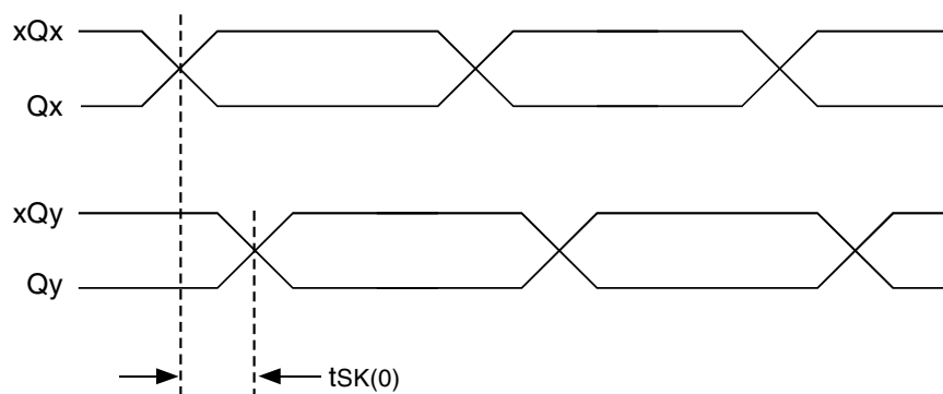
Output Skew
