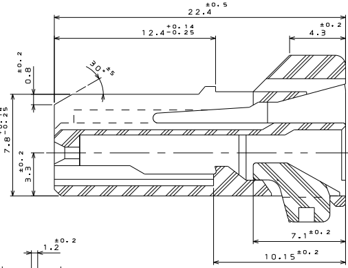
断面 A-A (尺度 5:1)
