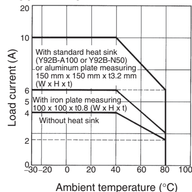
G3NA-D210B
