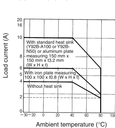
G3NA-440B
