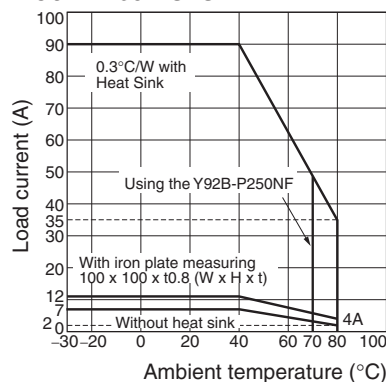
G3NA-290B-UTU-2 G3NA-490B-UTU-2
