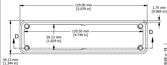
OPEN BEZEL
