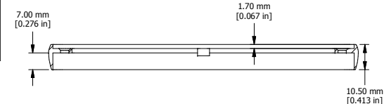
OPEN BEZEL
