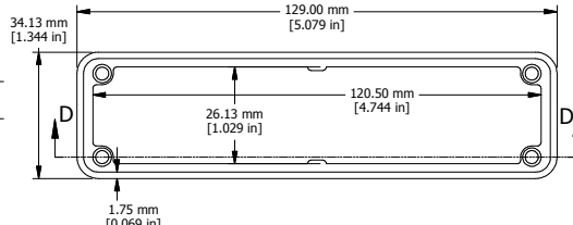
OPEN BEZEL
