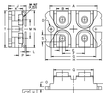
SOT-227B miniBLOC (IXGN)
