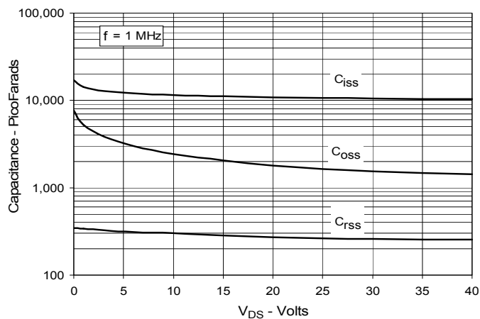
Fig. 11. Capacitance
