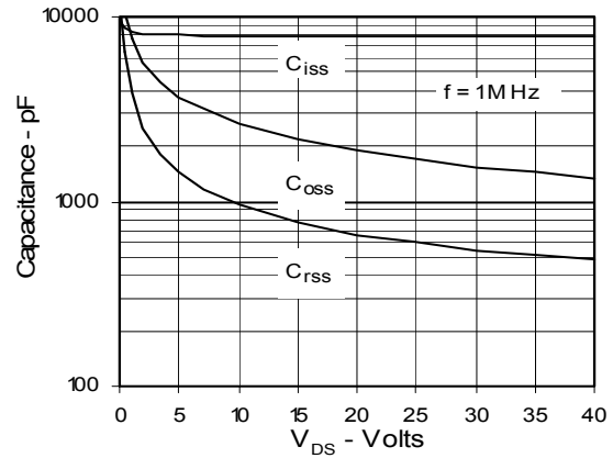
Fig. 10. Capacitance
