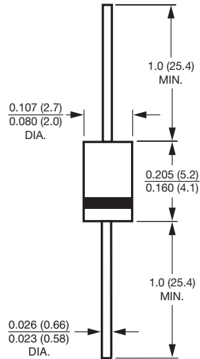
DO-204AL (DO-41)
